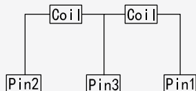
接线图（正磁钢）
